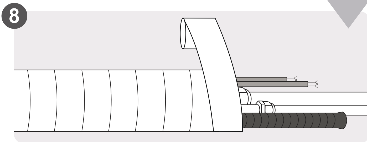
Izolacja rurek i przewodów (strona 18)
